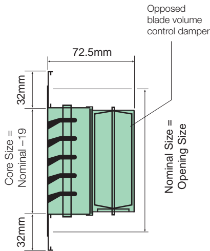
32W- NB15-R
